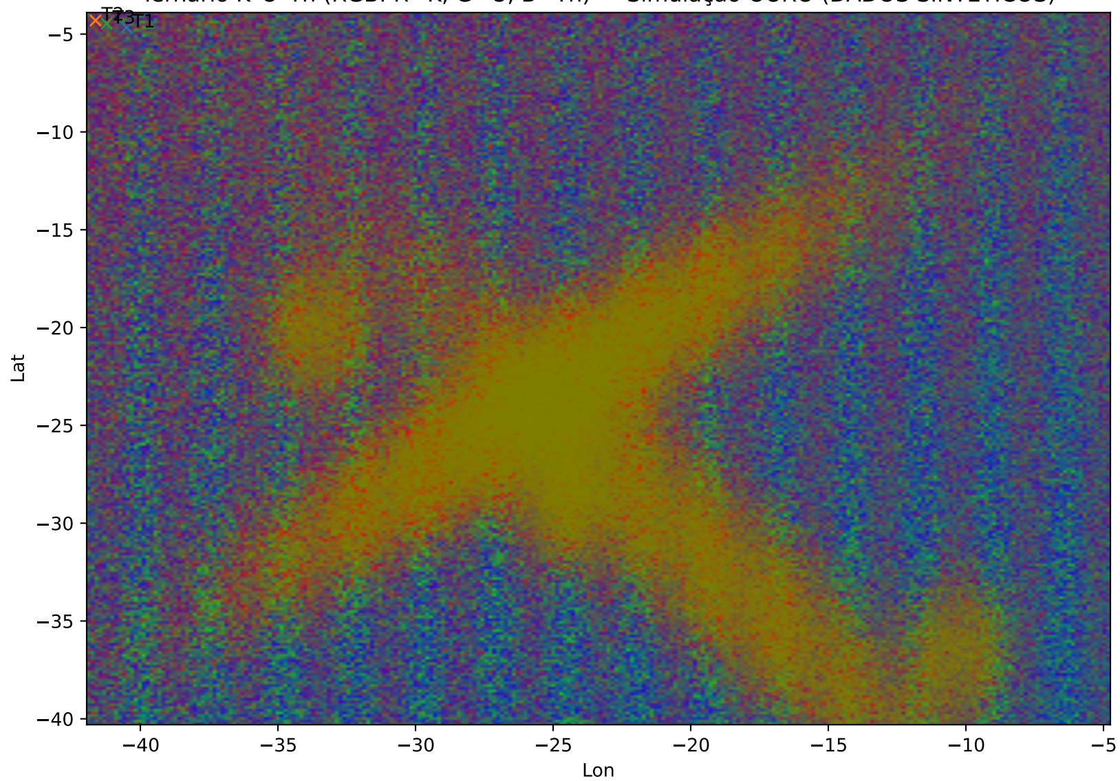
Ternário K-U-Th (RGB: R=K, G=U, B=Th) — Simulação OURO (DADOS SINTÉTICOS)
